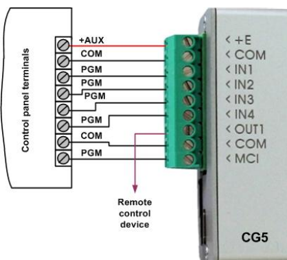
Paž.1. Bendroji jungimo prie apsaugos centralės schema, kai nustatytas nuolatinės jėjimų būsenų kontrolės režimas (24 h).
