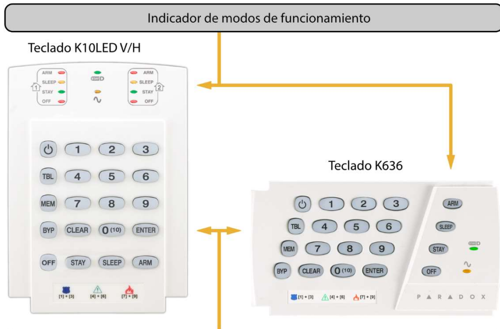
Botones retroiluminados para configurar modos de funcionamiento e ingresar números
