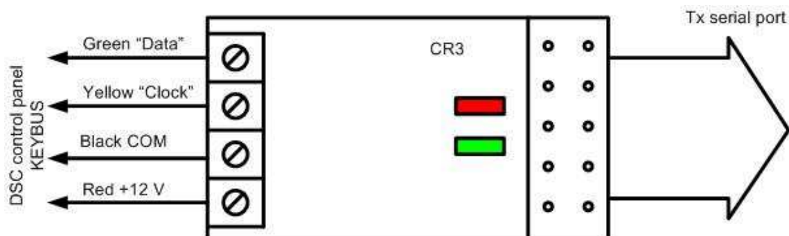
2 пр. Схема подключения CR3
