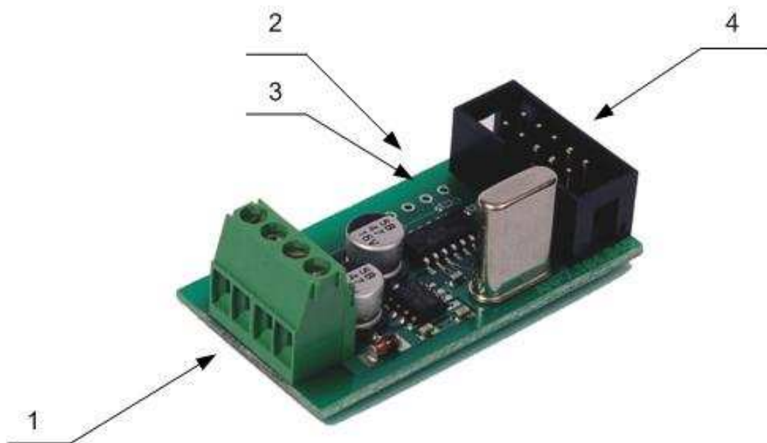
1 пр. Общий вид CR3
